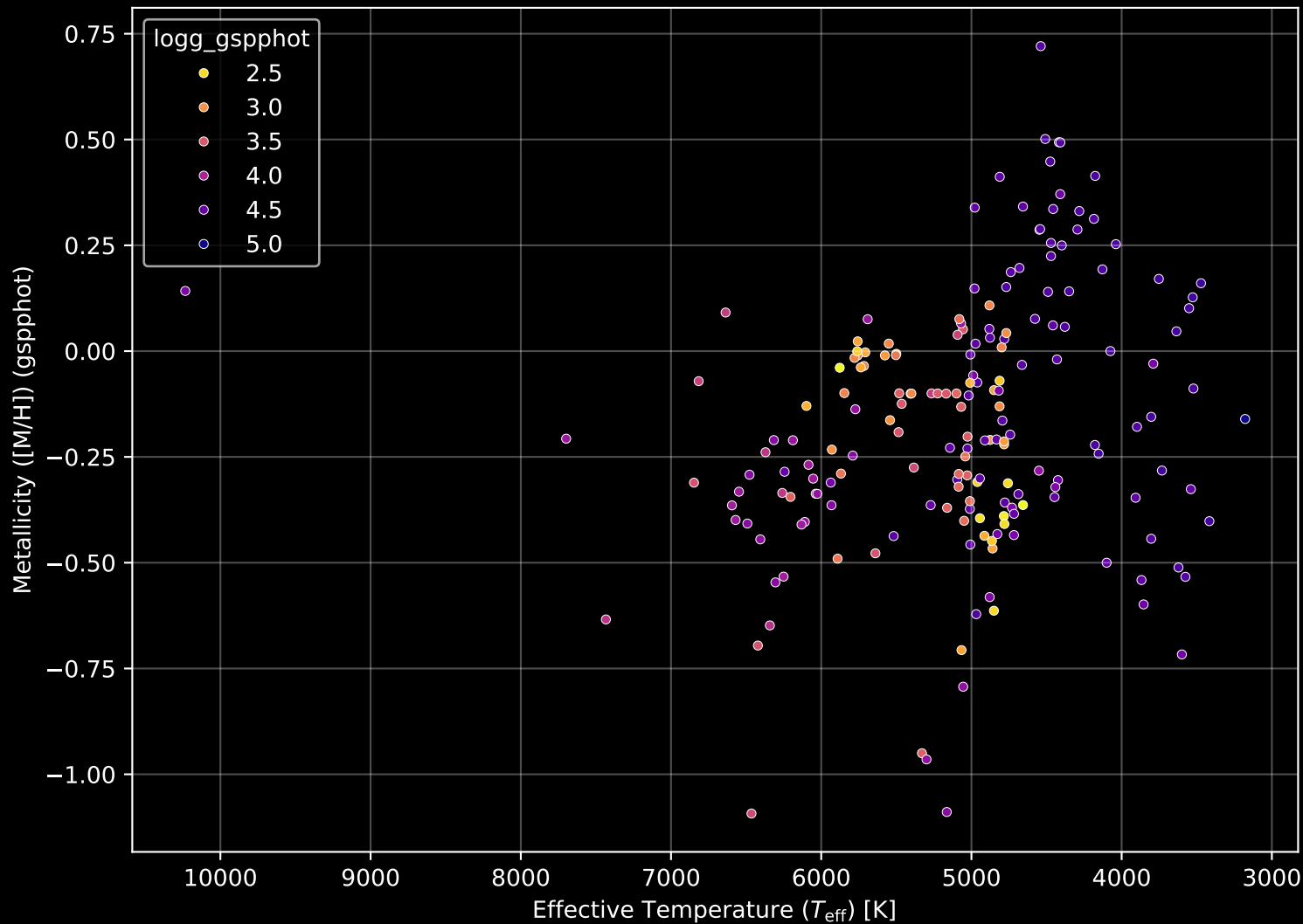
APOGEE DR17 Field: [280+60] Stellar Population Parameters (n= 190)
